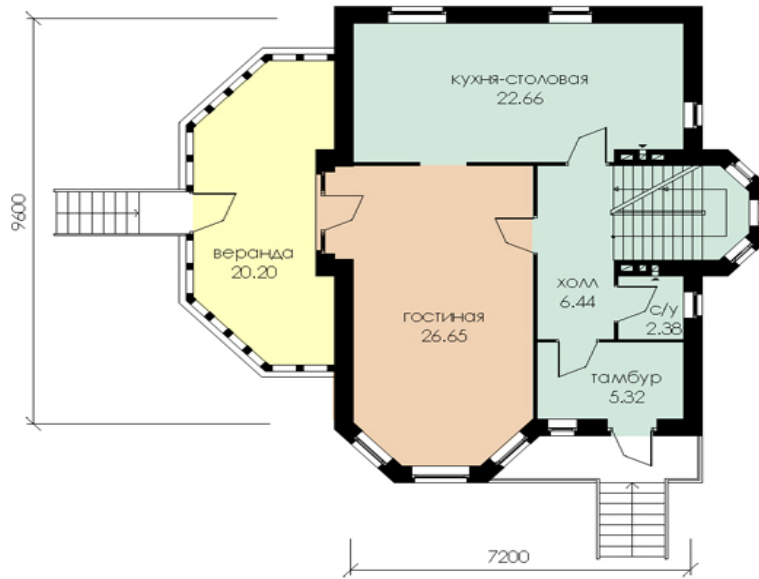
план I этажа
