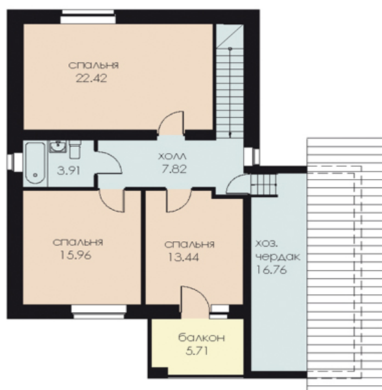
план 2 этажа
